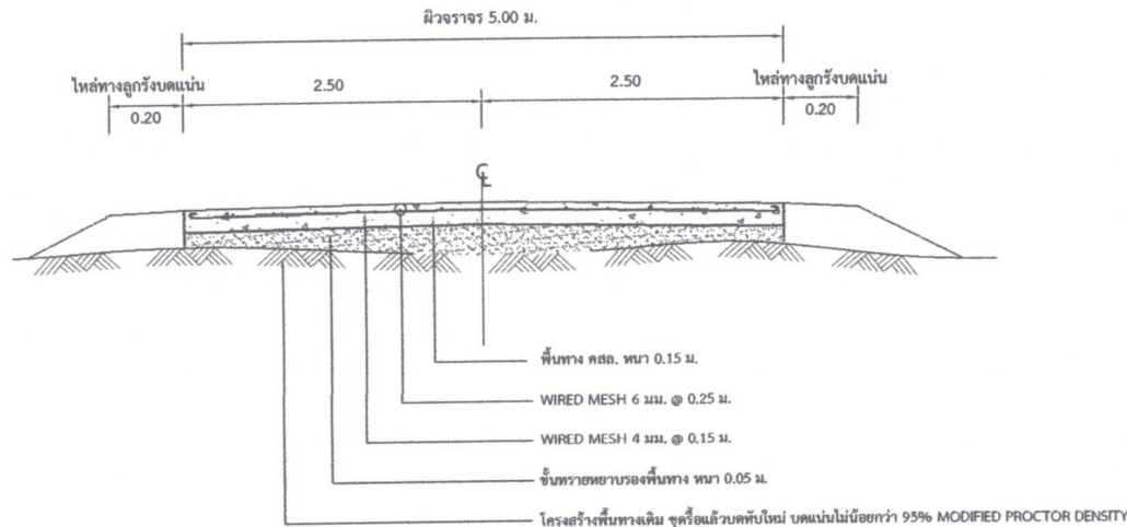
รูปตัดถนน คสล.
